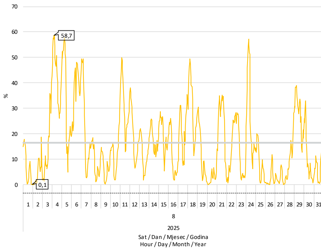
Slika 8 Udio proizvodnje vjetroelektrana u pokrivanju satnog opterećenja elektroenergetskog sustava u kolovozu 2025. godine
