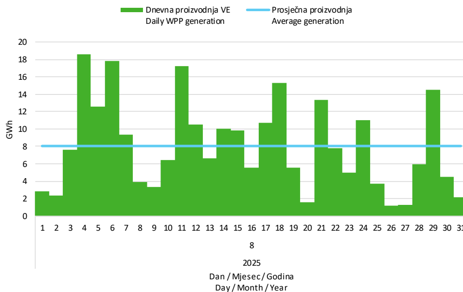
Slika 5 Dnevna proizvodnja svih vjetroelektrana u kolovozu 2025. godine
