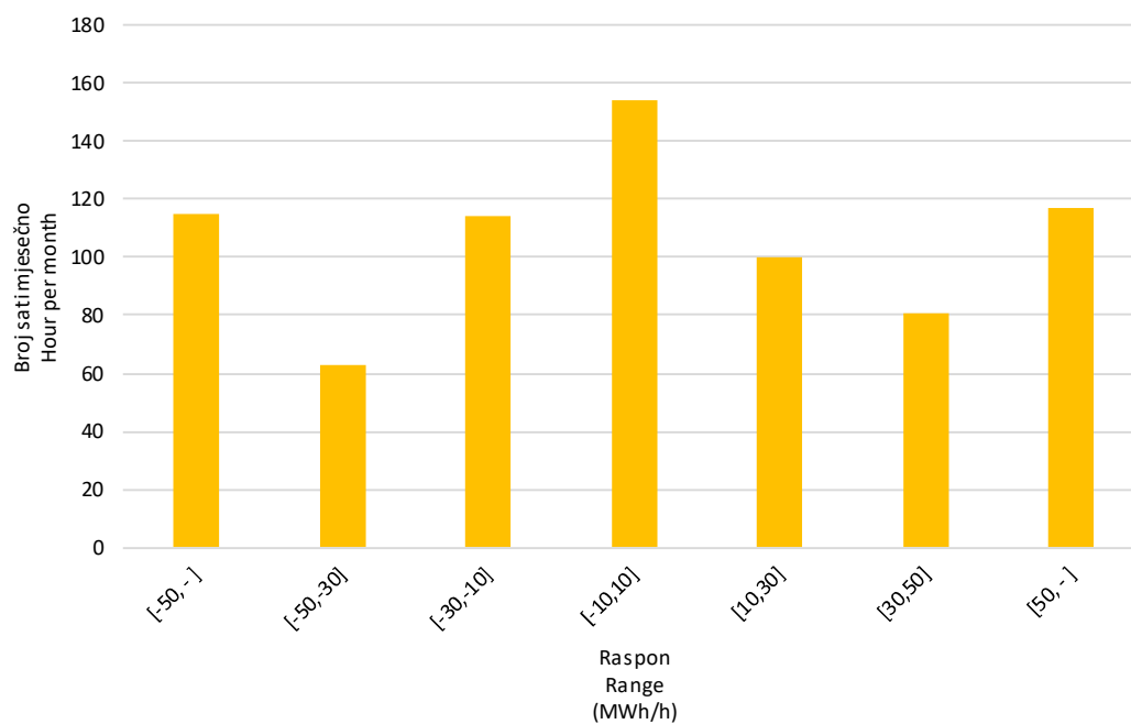
Slika 10 Statistička raspodjela satnih promjena proizvodnje VE u kolovozu 2025. godine
