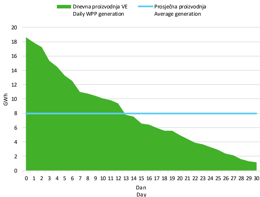
Slika 6 Krivulja trajanja dnevne proizvodnje vjetroelektrana u kolovozu 2025. godine
