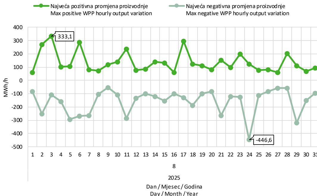
Slika 9 Maksimalna pozitivna i maksimalna negativna promjena satne proizvodnje VE u kolovozu 2025. godine
