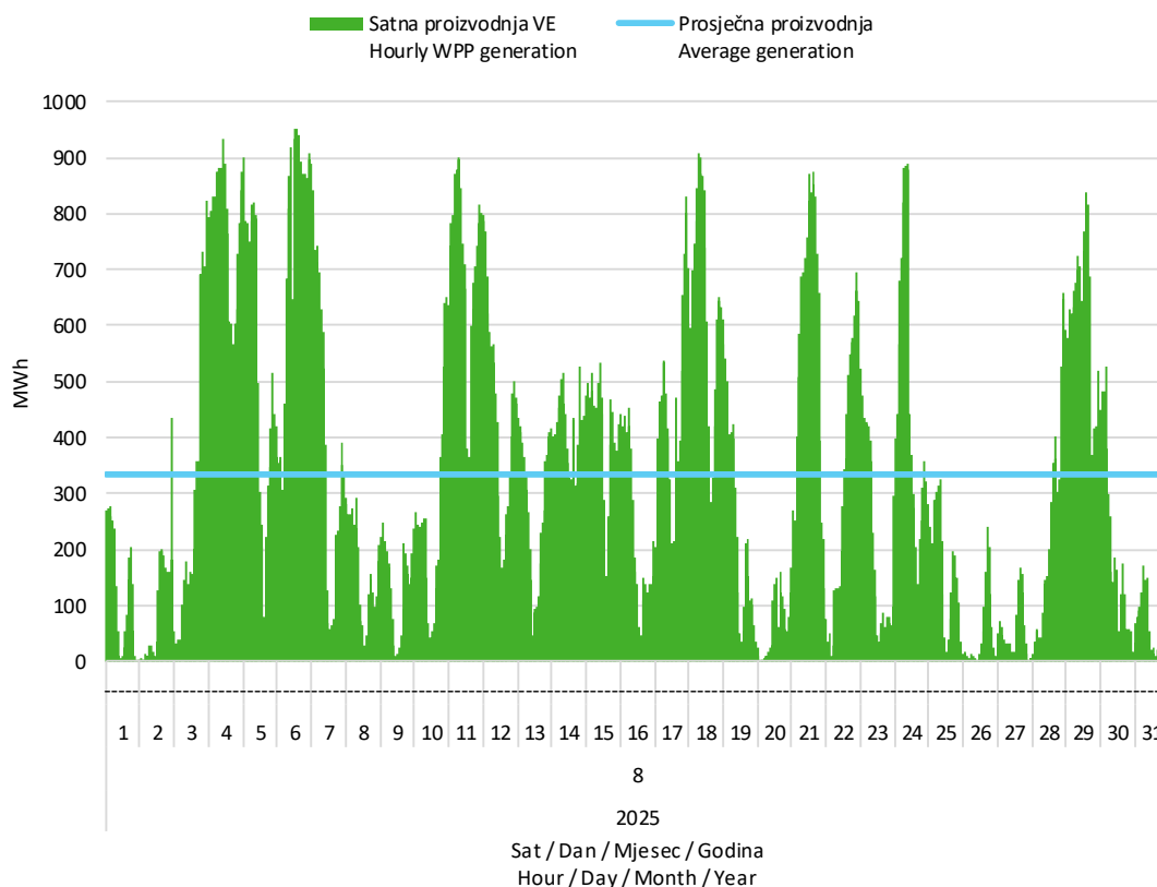
Slika 2 Satna proizvodnja svih vjetroelektrana u kolovozu 2025. godine
