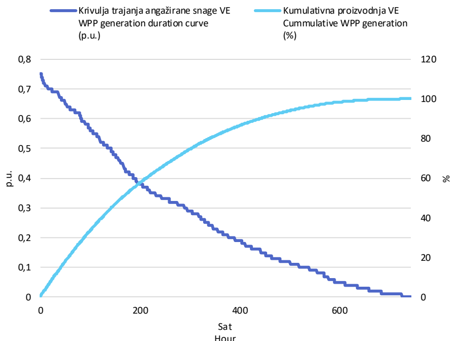
Slika 3 Krivulja trajanja angažirane snage svih VE i kumulativna proizvodnja VE u kolovozu 2025. godine u jediničnim vrijednostima
