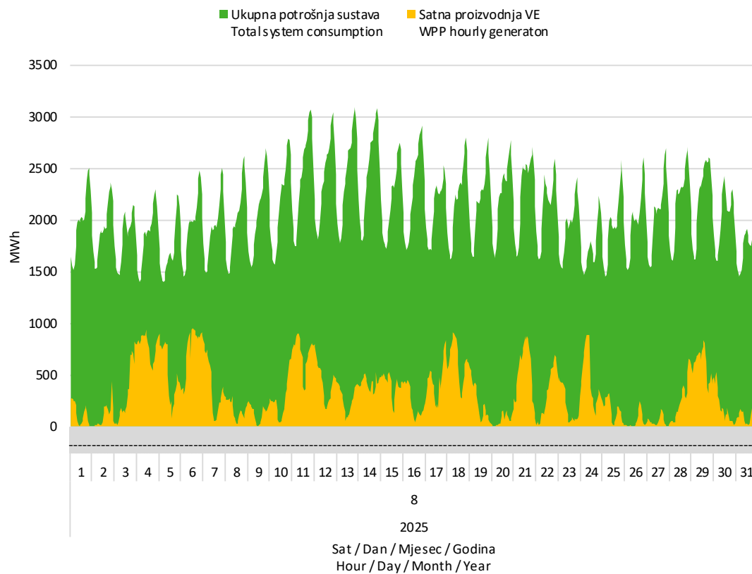
Slika 7 Usporedba satnog dijagrama opterećenja sustava i proizvodnje vjetroelektrana u kolovozu 2025. godine
